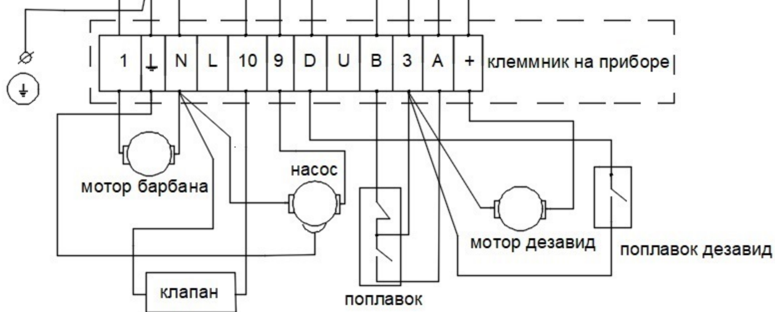
СХЕМА ЭЛЕКТРИЧЕСКАЯ МОНТАЖНАЯ FANLINE PRO-4005K-4805K-6005K
